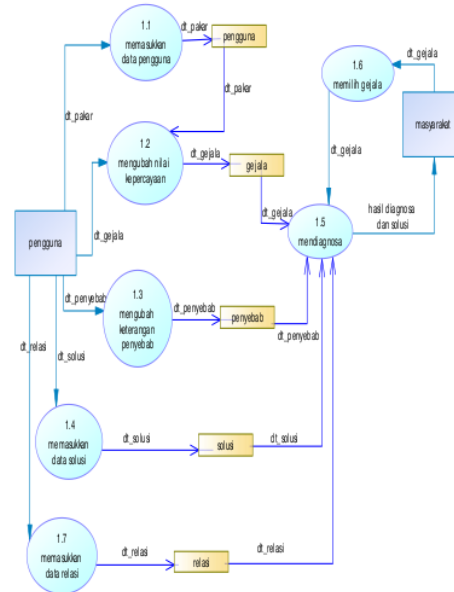
Gambar 4. Pemodelan Data Flow Diagram
