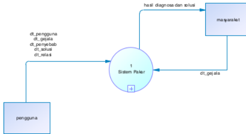
Gambar 3. Pemodelan Context Diagram
