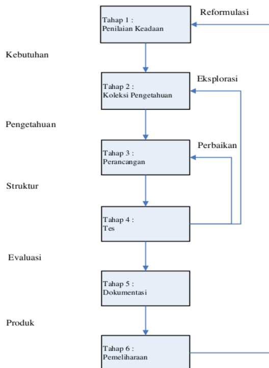
Gambar 1. Tahap-tahap Pengembangan Sistem Pakar
