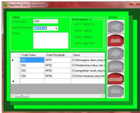
Gambar 10. Perancangan Form Data Solusi
