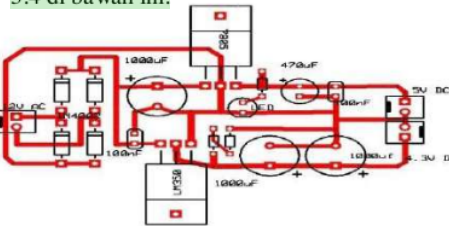
Gambar 3.4 Skema Rangkaian Regulator 7805 dan LM350
