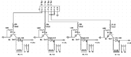
Gambar 3.5 Skema rangkaian relay
