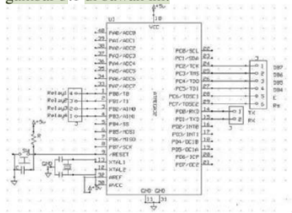
Gambar 3.1 Skema Rangkaian Sistem Minimum ATmega32L
