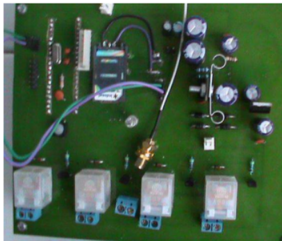
Gambar 3.6 Rangkaian Keseluruhan
