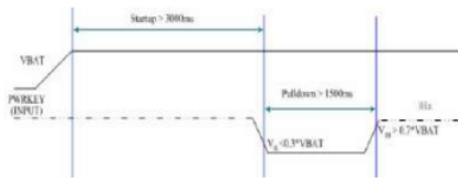
Gambar 2.1 Diagram waktu Powerkey untuk menyalakan SIM300CZ
