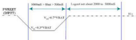
Gambar 2.2 Diagram waktu Powerkey untuk mematikan SIM300CZ
