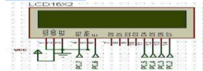
Gambar 3.3 Skema Rangkaian LCD 16x2
