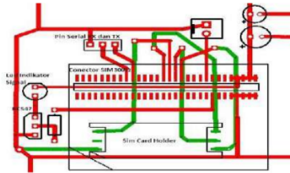
Gambar 3.2 Skema Rangkaian Modul Sim300cz
