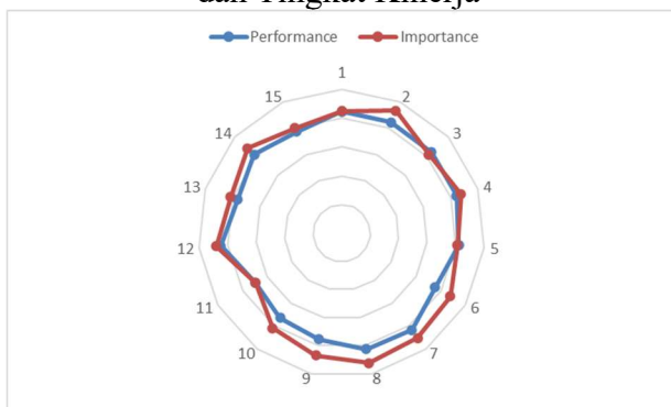
Gambar 3. Perbedaan Tingkat Kepentingan dan Tingkat Kinerja
