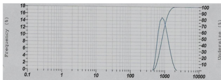
Gambar 1. Ukuran partikel nanoenkapsulasi
