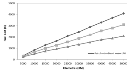
Gambar 1. Perbandingan Jarak Tempuh dan Biaya Bahan Bakar
