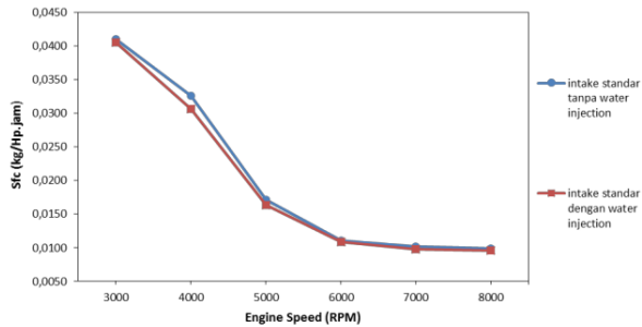
Gambar 6. Grafik Konsumsi Bahan Bakar Spesifik
