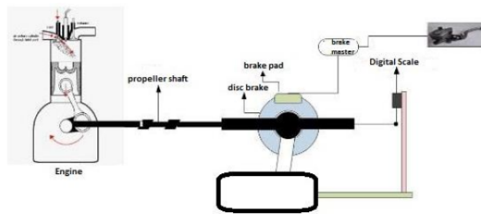
Gambar 5. Skema Pronybrake Dynamometer
