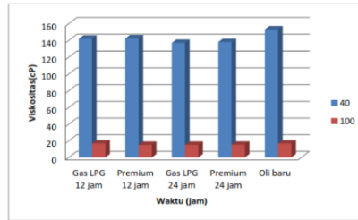
Gambar 2. Perbandingan Viskositas Oli Mesin
