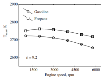
Gambar 3. Perbandingan Suhu Bahan Bakar LPG dan Gasoline
