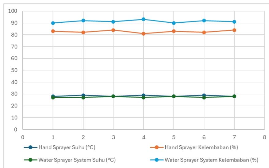
Gambar 6. Grafik Hasil pengukuran Suhu dan Kelembaban Kumbung
