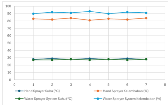
Gambar 6. Grafik Hasil pengukuran Suhu dan Kelembaban Kumbung
