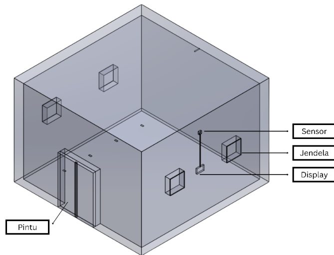
Gambar 1. Desain Kumbung Jamur Tiram
