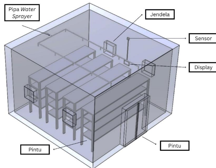
Gambar 5. Desain Kumbung Keseluruhan
