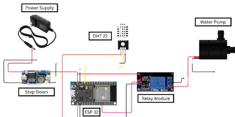
Gambar 4. Desain Skematik Sensor
