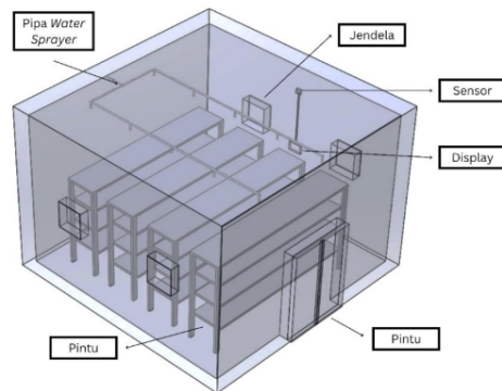
Gambar 5. Desain Kumbung keseluruhan
