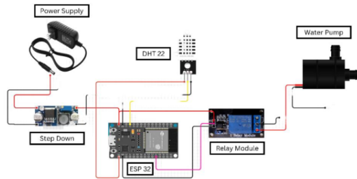
Gambar 4. Desain Skematik Sensor
