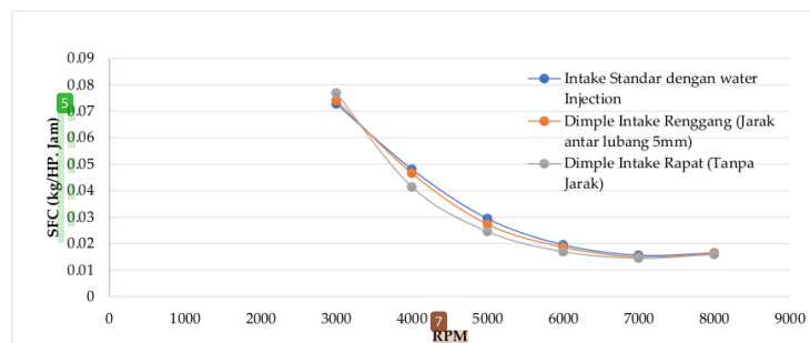
Gambar 4. Grafik perbandingan nilai SFC terhadap putaran mesin
