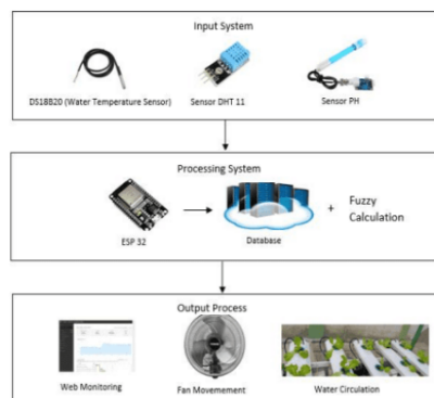
Gambar 1. Desain Sistem
