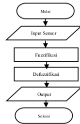
Gambar 3. Algoritma fuzzy
