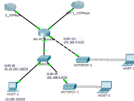
Gambar 2 Topologi Jaringan
