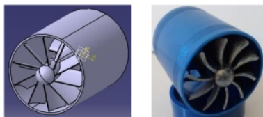
Gambar 2. Desain Fan Aksial
