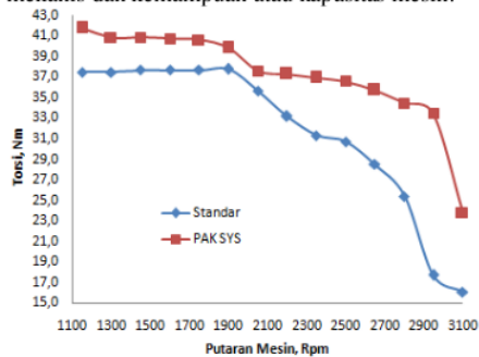
Gambar 5. Hubungan torsi terhadap variasi putaran mesin
