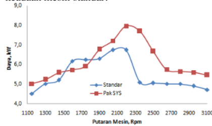
Gambar 6. Hubungan daya terhadap variasi putaran mesin
