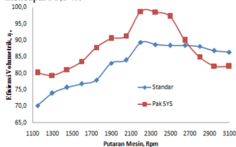
Gambar 7. Hubungan efisiensi volumetrik terhadap variasi putaran mesin
