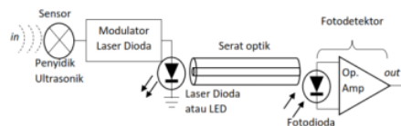
Gambar 3. Diagram blok sistem transmisi data menggunakan serat optik (Sumber: Waluyo dan Agus, 2009)
