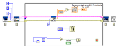
Gambar 8. Jendela block diagram LabVIEW untuk pembacaan tegangan keluaran Pada pembacaan tegangan keluaran rangkaian Op Amp digunakan simbol Analog Read Pin.vi . Adapun
