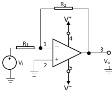
Gambar 4. Rangkaian penguat operasional
