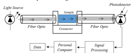
Gambar 5. Desain rangkaian alat ukur
