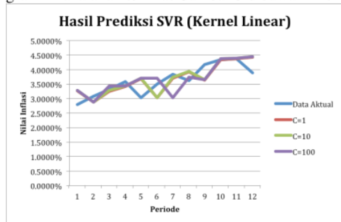
Gambar 5 Grafik perbandingan uji kernel linear
