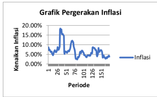
Gambar 4 Data inflasi periode Maret 2003 sampai dengan Juli 2017
