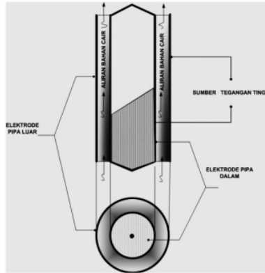
Gambar 4. Elektroda Pipa Koaksial
