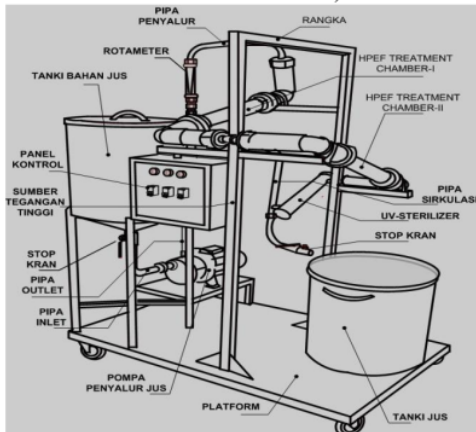
Gambar 3. Teknologi Pasteurisasi Minuman Yogurt Berbasis HPEF
