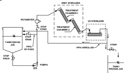
Gambar 2.4. Aliran Proses Sterilisasi
