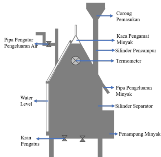
Gambar 1. Desain alat separator
