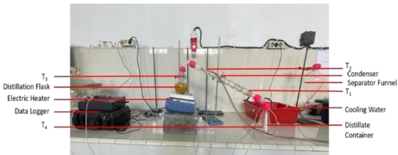
Gambar 1. Pemasangan alat distilasi
