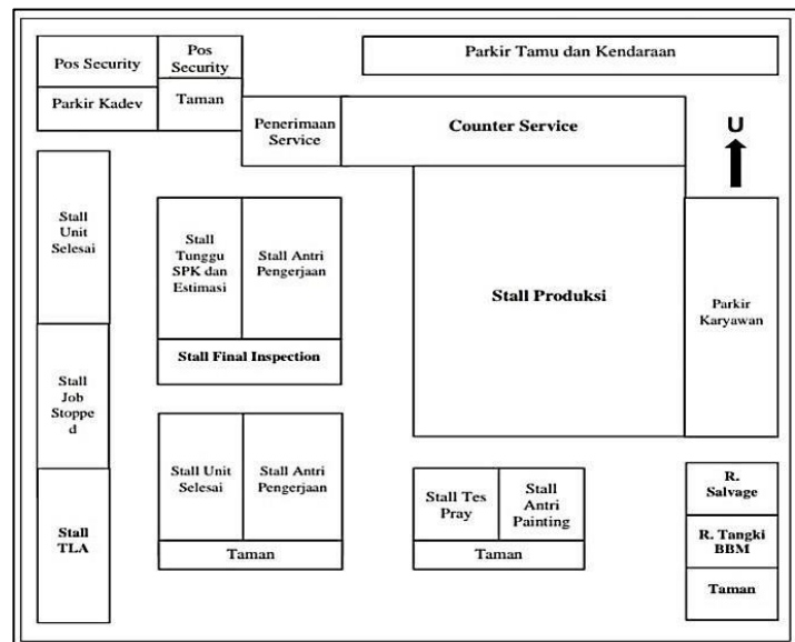
Gambar 1.2 Tata letak Auto 2000 BP Jember
