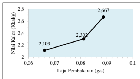
Gambar 5. Nilai Kalor vs Laju Pembakaran
