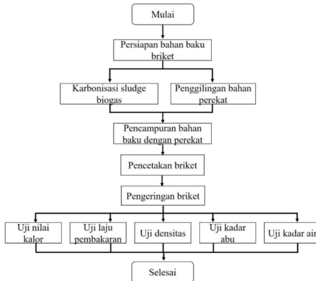
Gambar 3. Diagram Alir Pembuatan Briket
