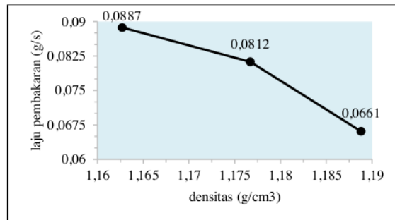
Gambar 7. Laju pembakaran vs densitas
