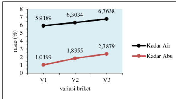
Gambar 8. Nilai Kadar air dan Kadar Abu
