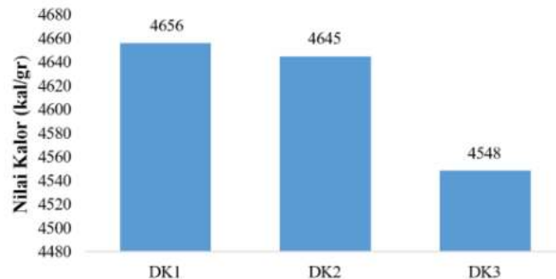
Gambar 9. Grafik Nilai Kalor Briket
