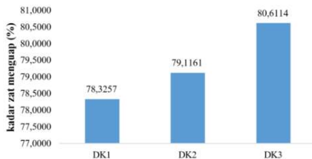
Gambar 6. Grafik Volatile Matter Briket
