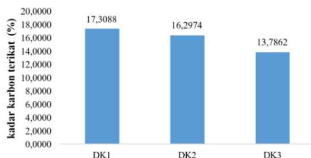
Gambar 7. Grafik Kadar Karbon Terikat Briket
