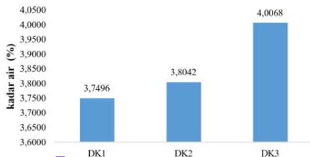
3 Gambar 4. Grafik Kadar Air Sampel Briket
