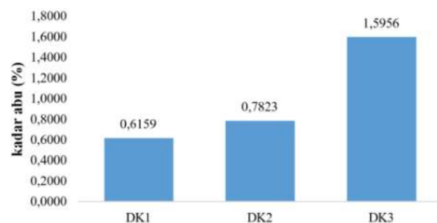
Gambar 8. Grafik Kadar Abu Briket
