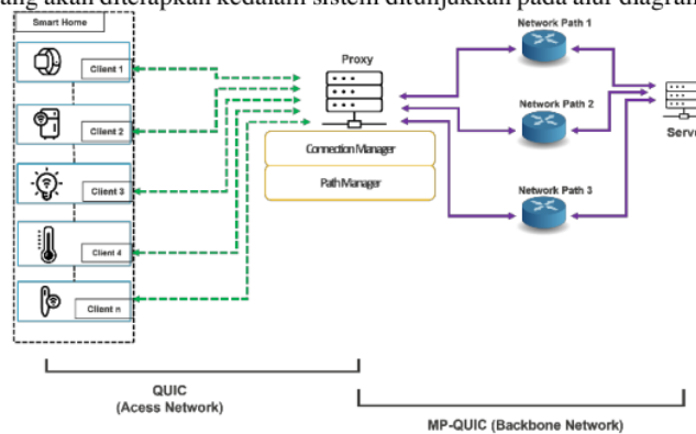
Gambar 2 Desain Sistem Jaringan
