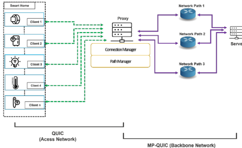
Gambar 1 Skema Jaringan Antara Client - Server
