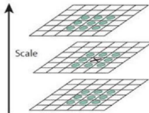
Gambar 4. Menentukan Titik Maxima dan Minima untuk Keypoint
