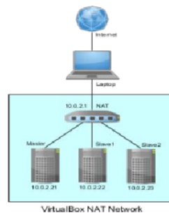
Gambar 1. Topologi jaringan NAT VirtualBox
