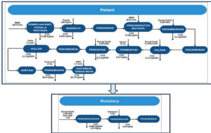
Gambar 3. Neraca energi rantai pasok kopi
