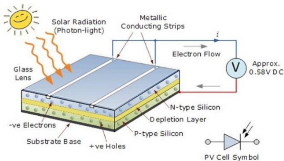
Gambar 4.1 Proses terjadinya fotovoltaiik pada sel surya
