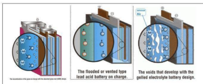
Gambar 3.13 Baterai VRLA Gel sumber: kosasih (2018)
