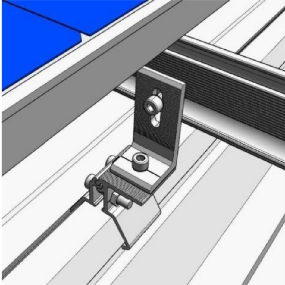
Gambar 4.28 pemasangan Kliplok dan L-feet (Sumber : Solaracks)
