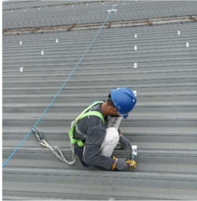
Gambar 4.33 Pemasangan Mounting Sistem (Sumber : ATW Solar)
