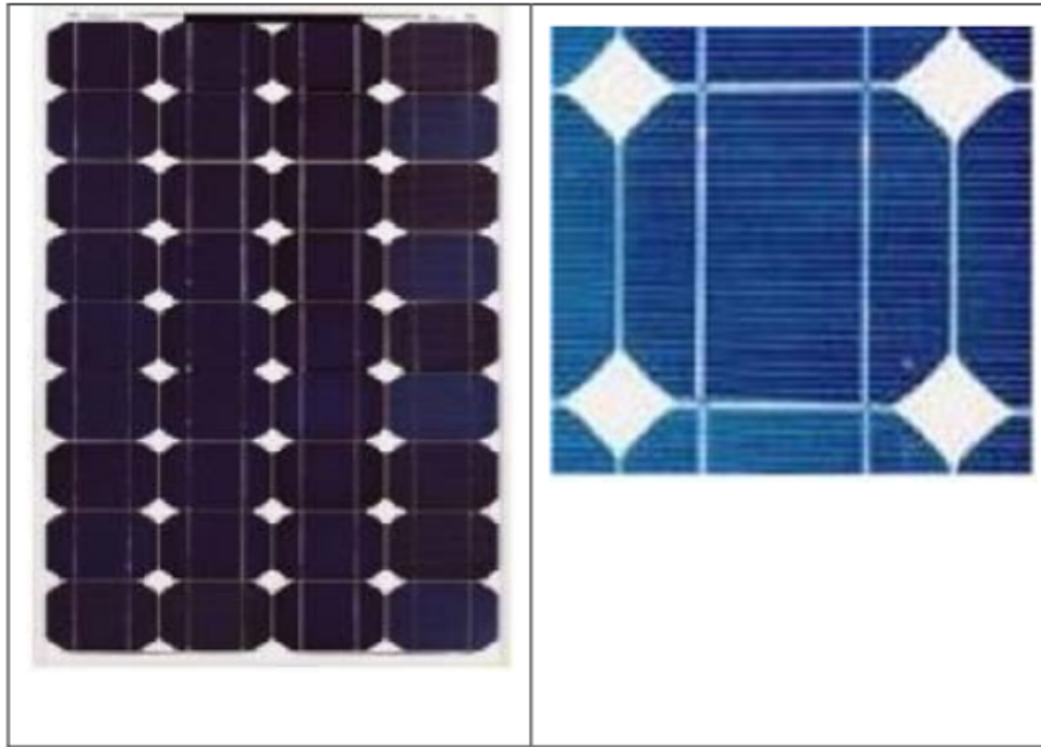
Gambar 3.5. Gambar Modul Surya Jenis Monokristalin
