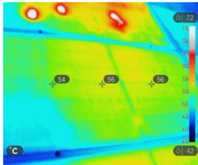
Gambar 5.6 Pengecekan Suhu Panel Surya Menggunakan Kamera Thermal (Sumber: data primer diolah 2022)
