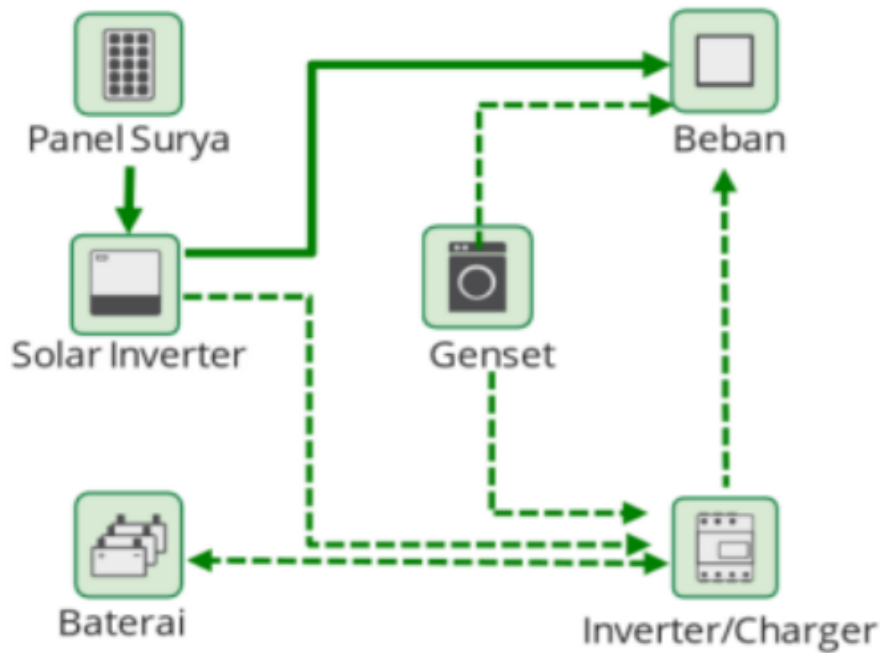
Gambar 4.9 Skema Sistem Hybrid
