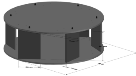
Gambar 1. Model 3D Tampak Keseluruhan Pada Sudut Kemiringan 40°
