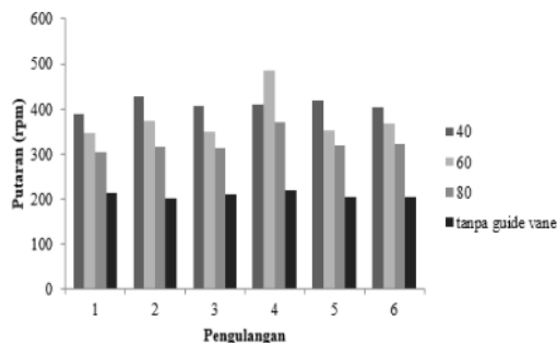
Gambar 7. Grafik Pengaruh Putaran Angin Tanpa Beban pada Jarak 150 cm
