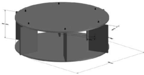
Gambar 3. Model 3D Tampak Keseluruhan Pada Sudut Kemiringan 80°
