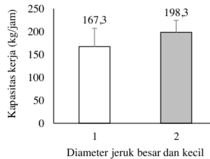
Gambar 4. Kapasitas kerja mesin pembelah dan pemereras jeruk manis Semboro besar Ø 65 mm (□) dan jeruk kecil Ø 49 mm (■)
