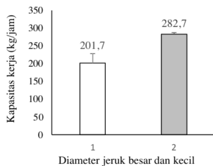
Gambar 6. Kapasitas kerja mesin pembelah dan pemas jeruk manis Semboro besar \varnothing 65 mm (□) dan jeruk kecil \varnothing 49 mm (■)
