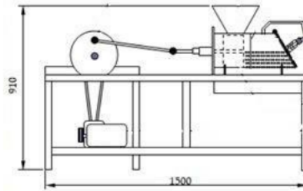
Gambar 1. Desain mesin pembelah dan pemas jeruk manis
