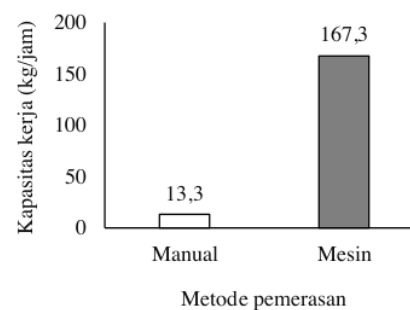
Gambar 8. Nilai perbandingan kapasitas kerja pemerasan dengan manual/tangan (□) dan mesin pembelah dan pemas jeruk manis Semboro (■)
