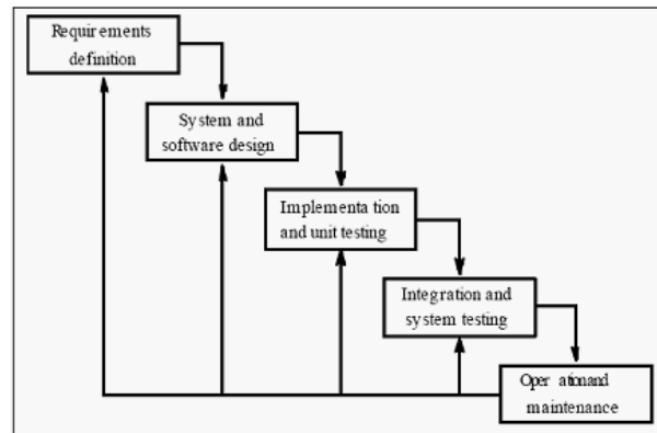
Gambar 1.2 Waterfall menurut Sommerville
