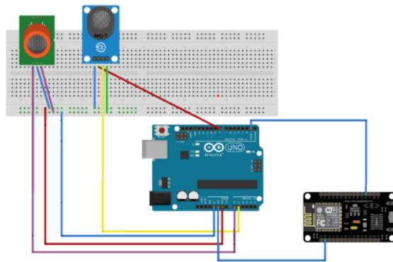
Gambar 6. Skema Rangkaian
