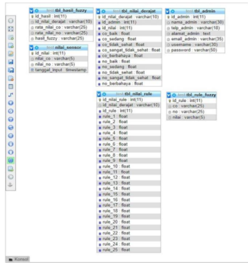
Gambar 12. Implementasi Database
