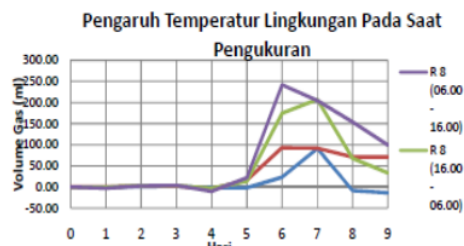
Gambar 4.4 Grafik Perbandingan Produksi Biogasi Dalam Ruangan dan Luar Ruangan [6].
