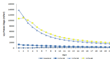
Grafik 4.2 Laju Produksi Biogas
