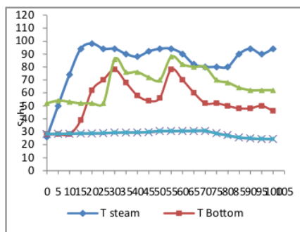
GAMBAR 2. GRAFIK SEBARAN SUHU PADA PROSES DIETILASI
