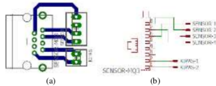
Gambar 3a. Layout Rangkaian Sensor MQ3; Gambar 3b. Skematik Rangkaian Sensor MQ3
