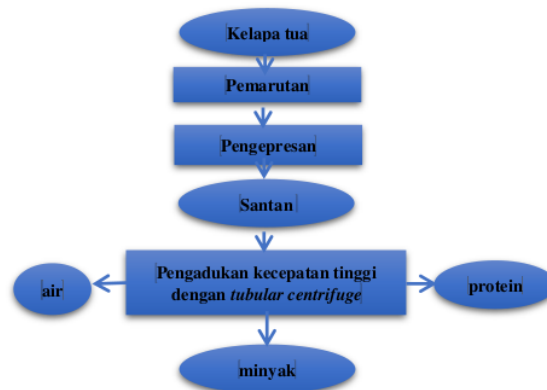
Gambar 1. Diagram alir pembuatan VCO
