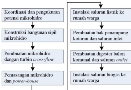
Gambar 3. Diagram alir kegiatan PTDM
