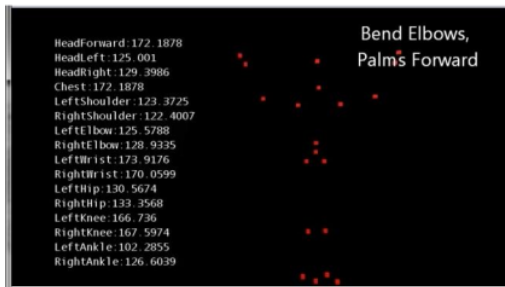
Gambar 7 Contoh perhitungan sudut pada pose gerakan fleksi
