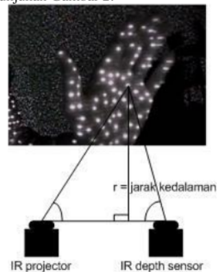
Gambar 2 Ilustrasi perhitungan kedalaman citra menggunakan Microsoft Kinect
