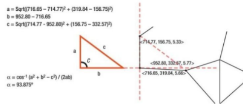
Gambar 6 Perhitungan sudut antara dua joint
