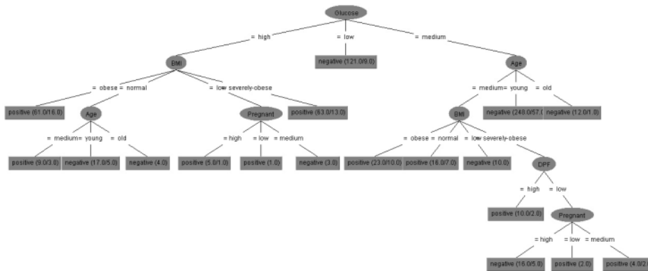
Gambar 2: Decision tree J48 pada diagnosis diabetes untuk dataset Pima Indians
