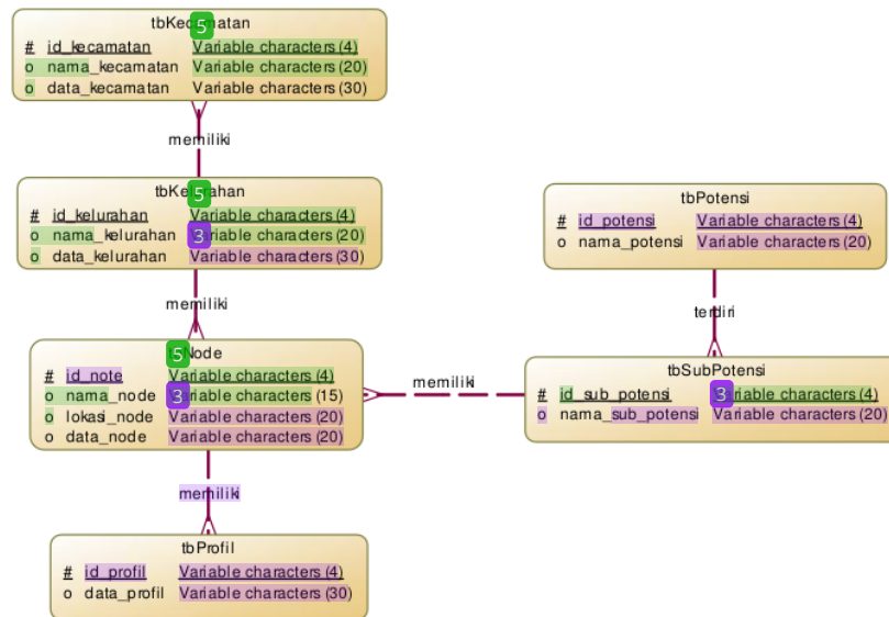
Gambar 2. Rancangan basis data sistem SoH
