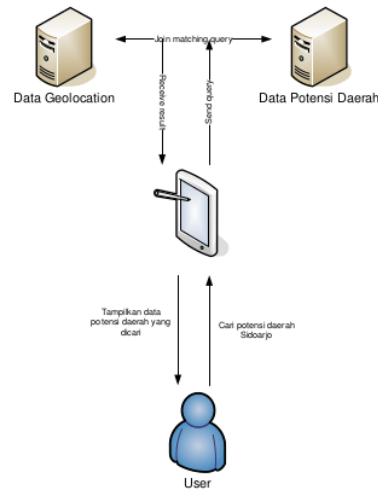
Gambar 1. Arsitektur SoH
