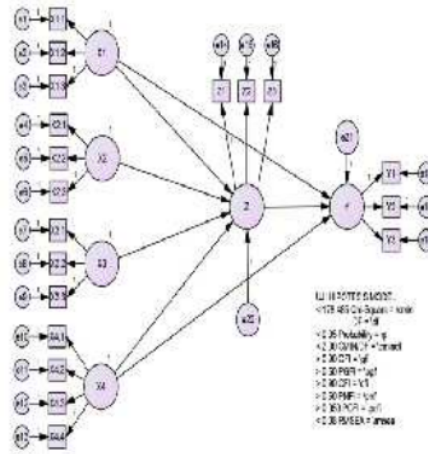
GAMBAR 2.FORMULASI MODEL SEM
