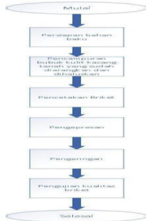
Gambar 2. Diagram Alir Pembuatan Briket
