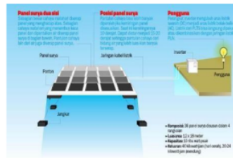
Gambar 2. Sistem Cara Kerja PLTS Terapung
