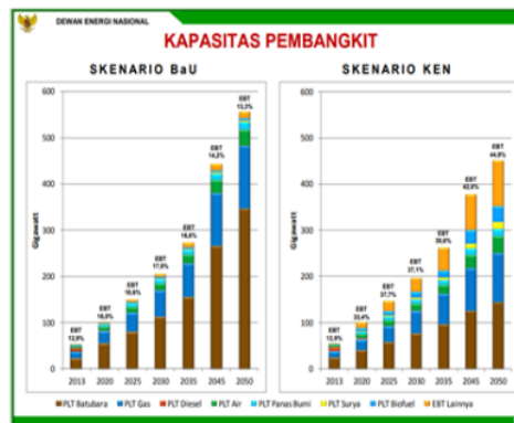
Gambar 1. Grafik kapasitas pembangkit Sumber: Dewan Energi Nasional 2014
