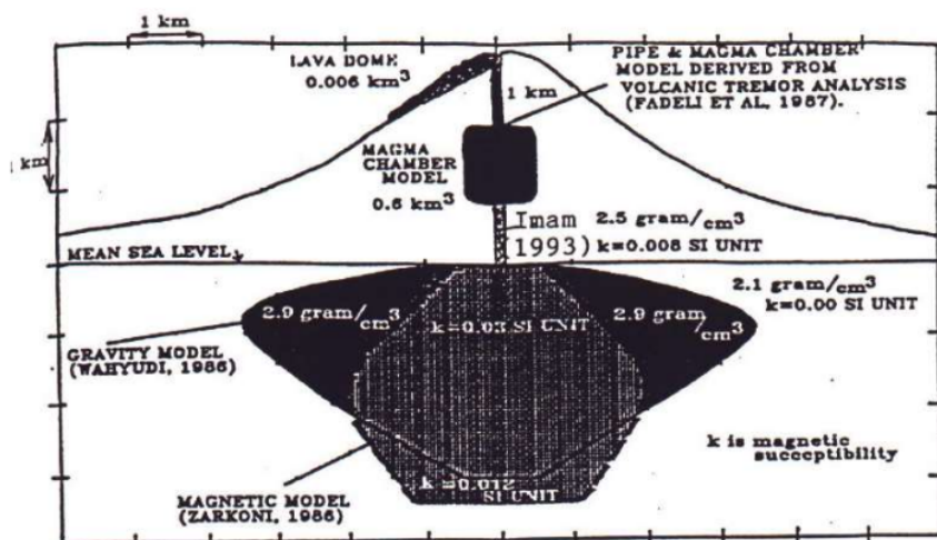
1 Gambar 10 Hasil interpretasi bawah permukaan Gunung Merapi dari beberapa macam metode. (Sumber: Suyanto, 2012)
