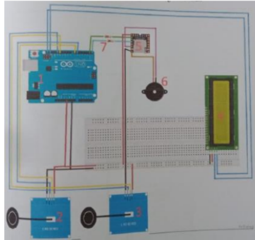
Gambar 4. Desain wiring alat bantu parker mobil
