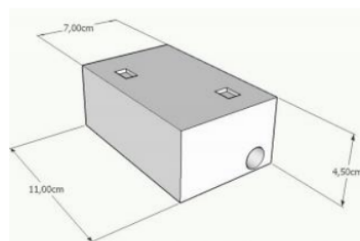
Gambar 3. Desain kotak komponen
