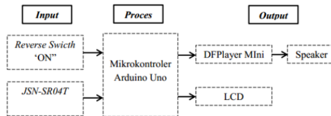
Gambar 1. Blok diagram sistem alat bantu parkir mobil
