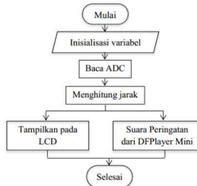
Gambar 2. Flowchart pembuatan program pada arduino uno
