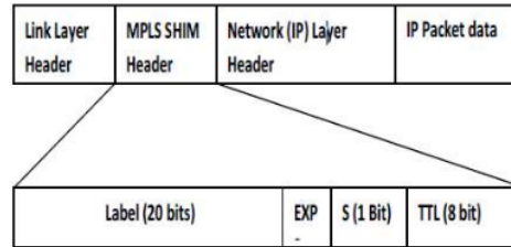
Gambar 1. MPLS Shim Header[9]
