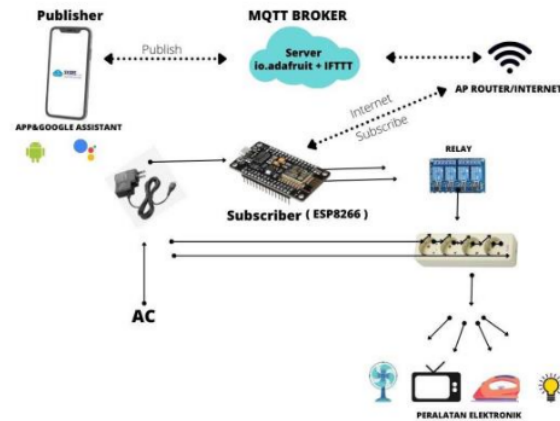
Gambar 2. Diagram blok sistem yang dikembangkan
