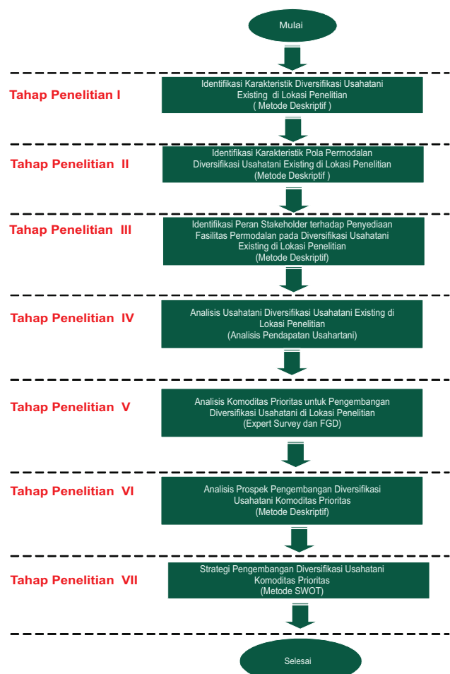
Gambar 1. Tahapan Penelitian
