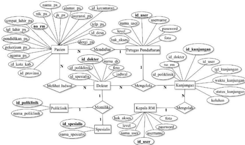
Gambar 9. ERD Sistem Pendaftaran Online Rawat Jalan
