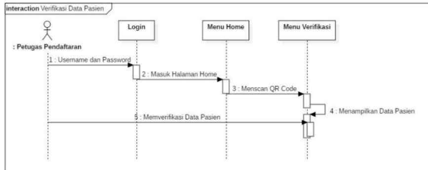
Gambar 7. Sequence Diagram Verifikasi Data Pasien
