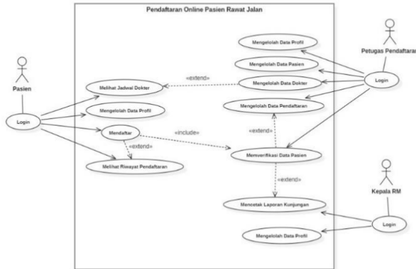
Gambar 2. Use Case Pendaftaran Online Pasien Rawat Jalan
