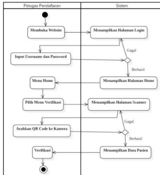
Gambar 4. Activity Diagram Verifikasi Data Pasien
