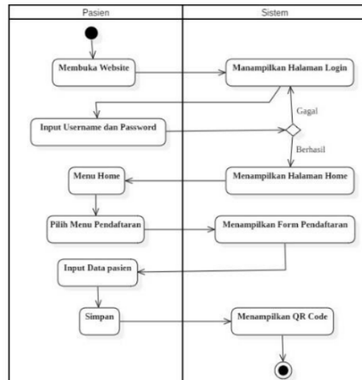
Gambar 3. Activity Diagram Pendaftaran Online Pasien Rawat Jalan
