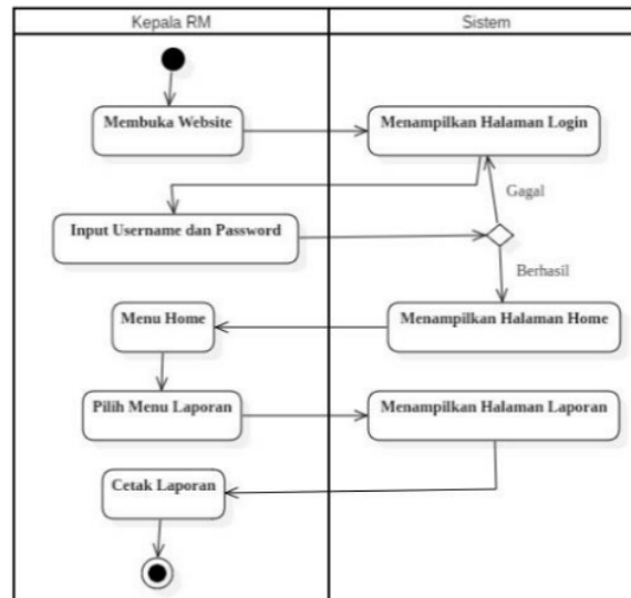
Gambar 5. Activity Diagram Laporan Kunjungan Pasien Rawat Jalan
