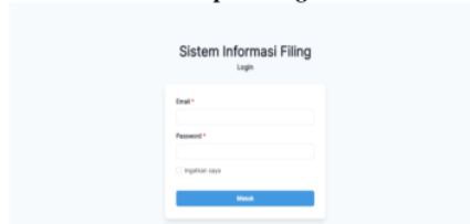
Gambar 8. Halaman Login
