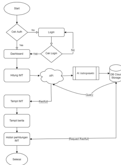
Gambar 1 Flowchart Aplikasi
