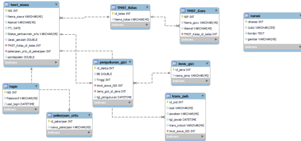
Gambar 3 desain database
