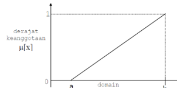
Gambar 2. Representasi Linear Naik (Kusumadewi dan Purnomo, 2004)
