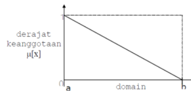
Gambar 3. Representasi Linear Turun (Kusumadewi dan Purnomo, 2004)
