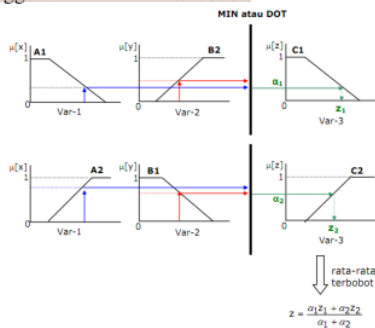
Gambar 6. Inferensi dengan menggunakan Metode Tsukamoto
