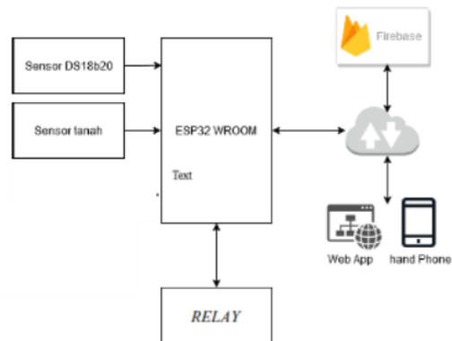
Gambar 1 Rancangan sistem monitoring suhu dan pengairan otomatis
