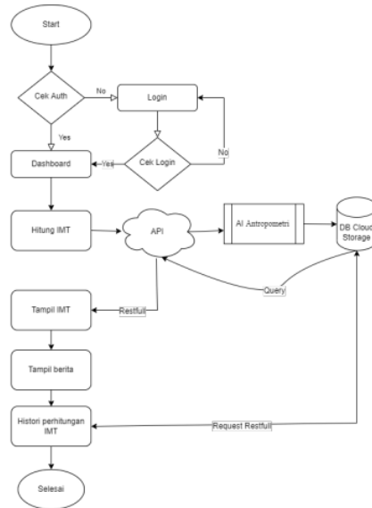
Gambar 1 Flowchart Aplikasi
