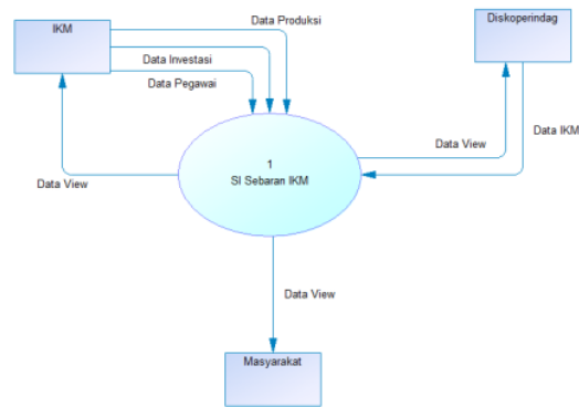
Gbr. 6 Diagram Konteks Sistem Informasi Sebaran IKM
